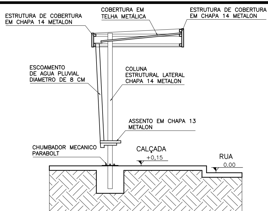
3 DETALHAMENTO 03 Escala 1:50
