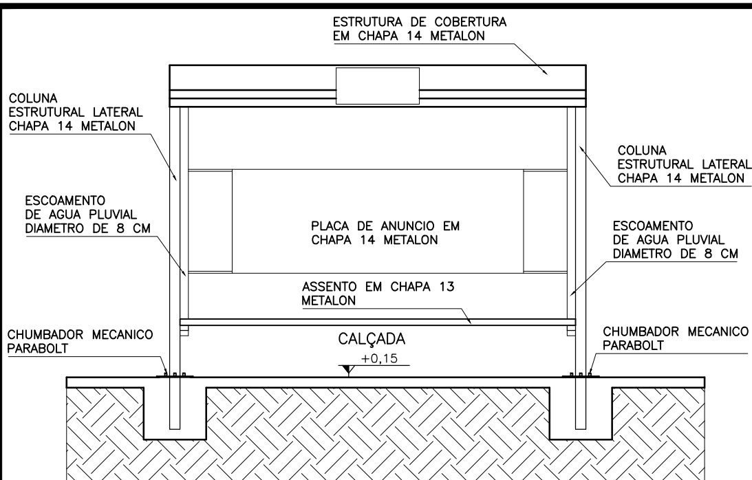
1 DETALHAMENTO 01 Escala 1:50
