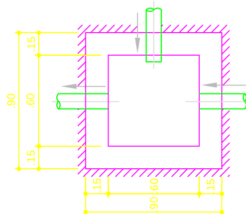
CAIXA DE INSPEÇÃO DE ESGOTO - 60x60 cm
