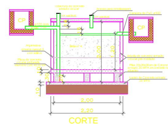
FILTRO ANAERÓBIO 2 M DE PROFUNDIDADE
