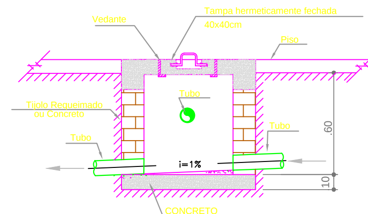
CAIXA DE INSPEÇÃO DE ESGOTO - 60x60 cm
