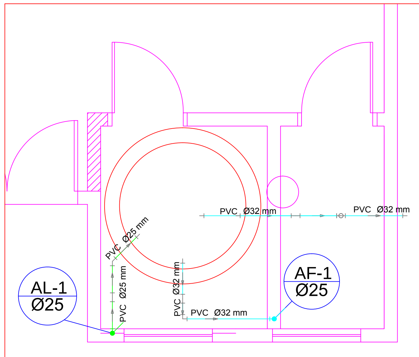
DET - 3
