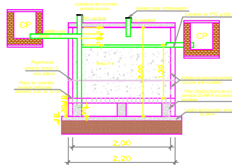
5 CORTE FILTRO ANAERÓBICO SEM ESCALA
