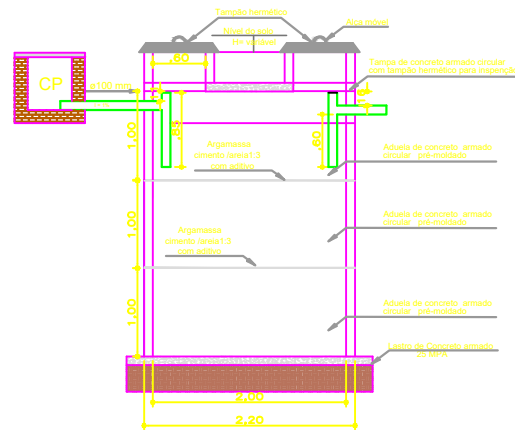
4 CORTE TANQUE SÉPTICO SEM ESCALA
